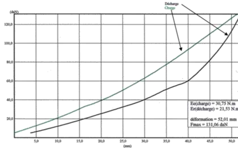
Figure 4 : courbe force/déformation, calcul de l'énergie
